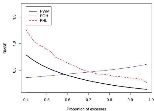
(d) RMSE for Burr(10, \frac{1}{4} ) model, n = 1000
