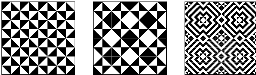
(a) Deux autres exemples de pavages réalisés par le Père TRUCHET vers 1704
