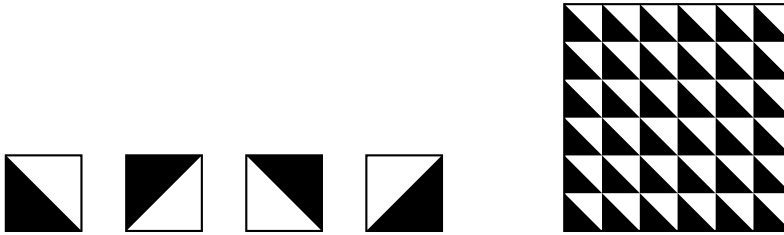
(a) Les quatre orientations possibles de la tuile utilisée par le Père TRUCHET
