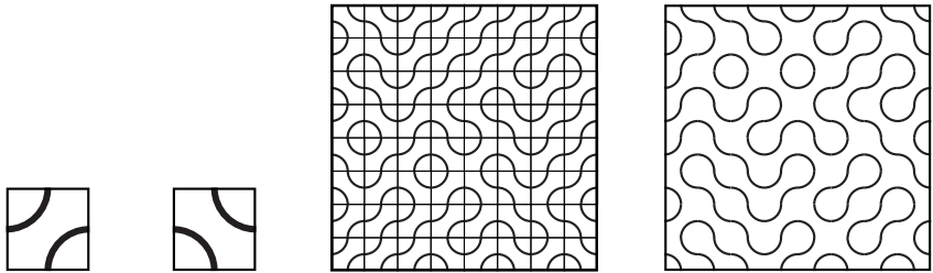
(a) Les deux orientations possibles de la tuile du pavage « à la TRUCHET » SLPT
