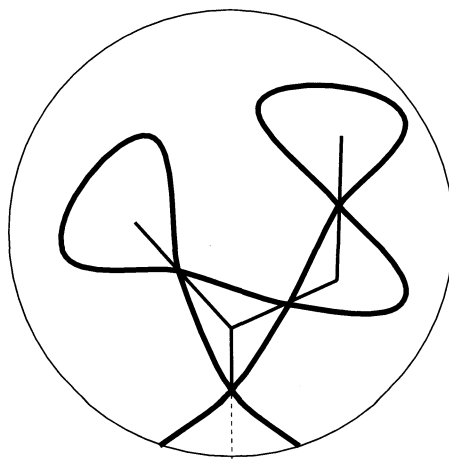
FIG. 2. - The slalom E_8
