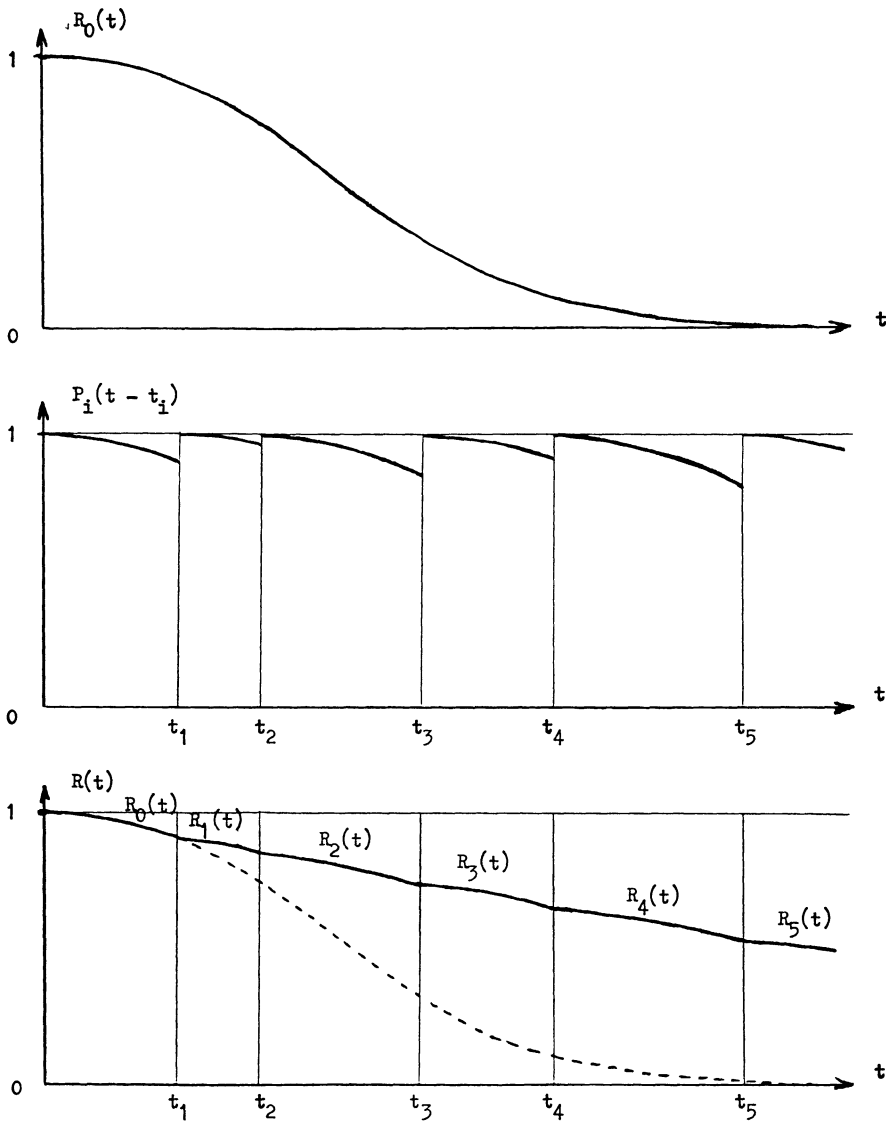
Figure 1. – La maintenance préventive permet de connaître l'état de chacun des éléments en redondance, et de réparer ceux qui sont défectueux. Le taux de défaillance de chacun des composants est constant.
